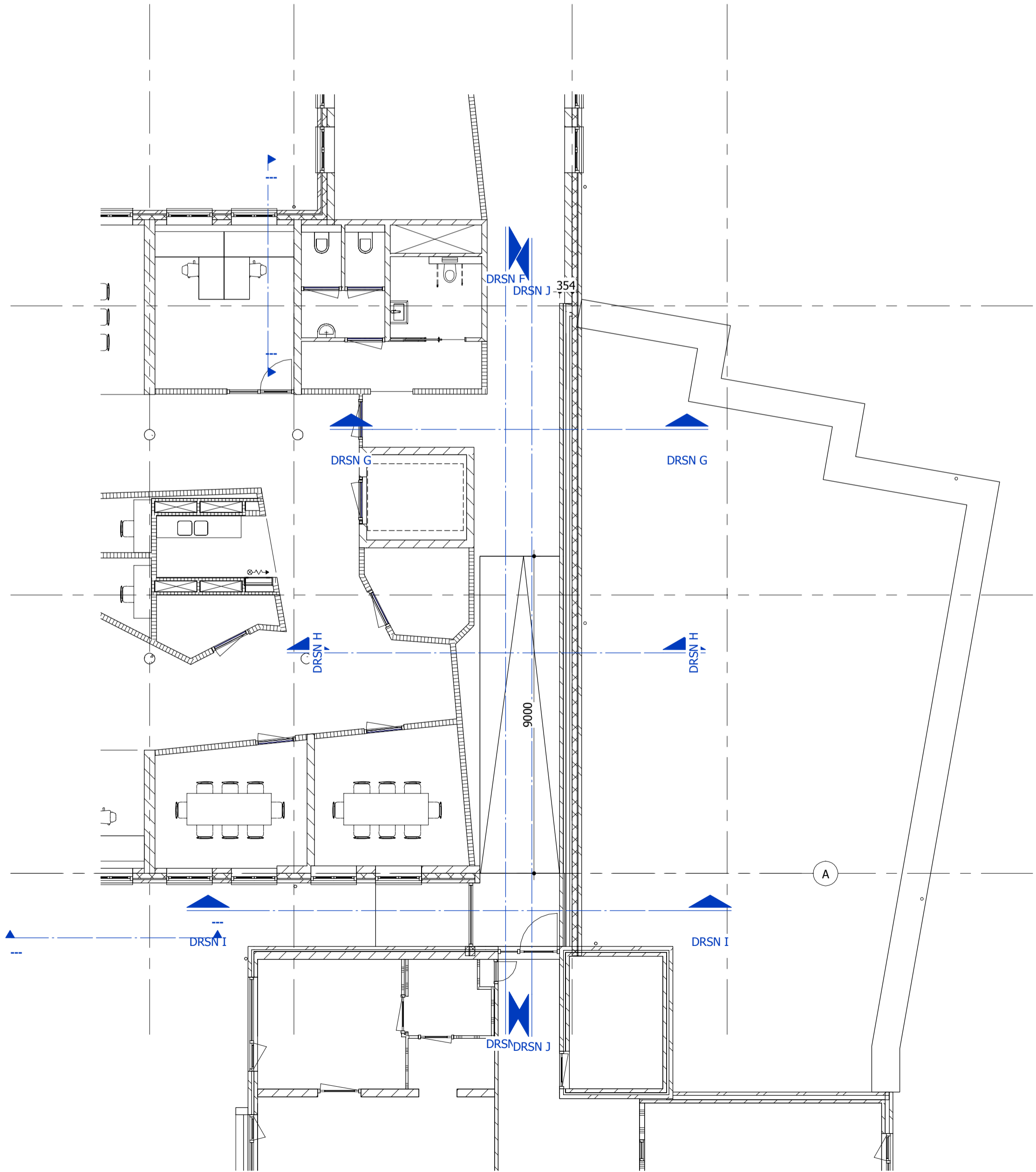
1e verdieping
